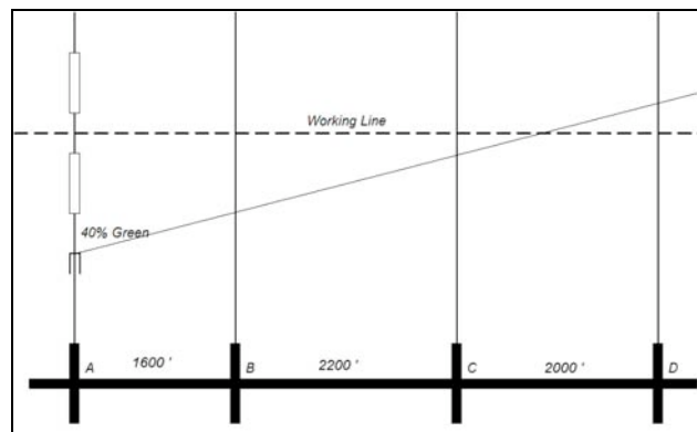
Figure . Kell Method (Beginning)
